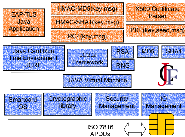
Figure 4 : Architecture java de la carte EAP-TLS
