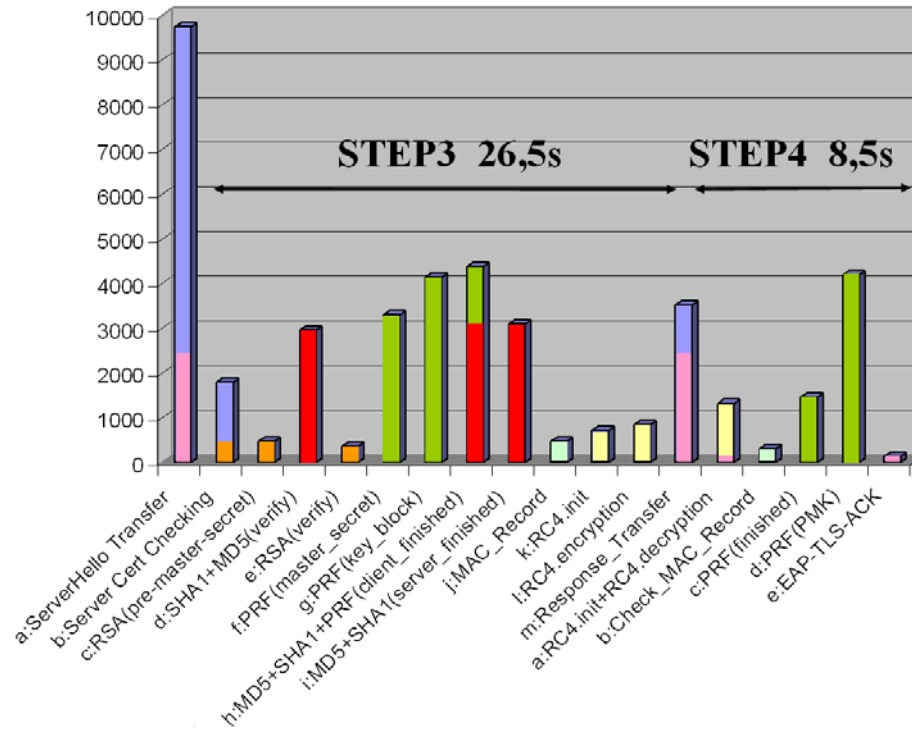
Figure 6: Exemple de répartition des temps calculs dans une carte EAP-TLS
