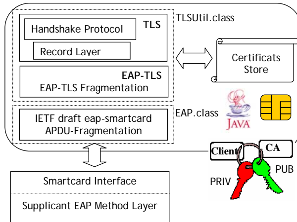
Figure 3 : La carte EAP-TLS
