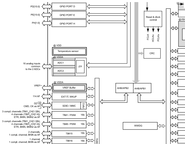
Microcontrôleur (issu du datasheet stm32l475xx )
