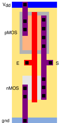
Layout d'un inverseur
