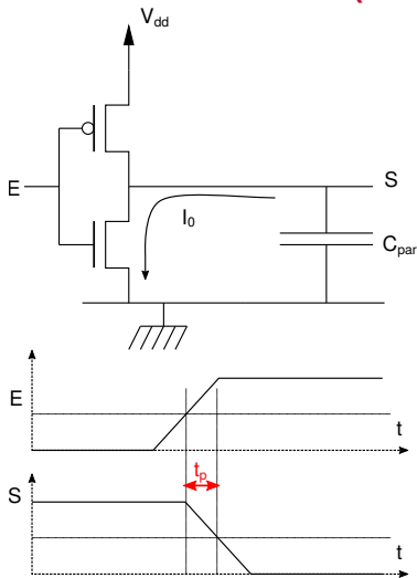
Temps de propagation d'une porte CMOS
