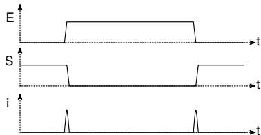
Consommation d'une porte CMOS
