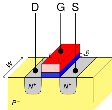
nMOS : dimensions
