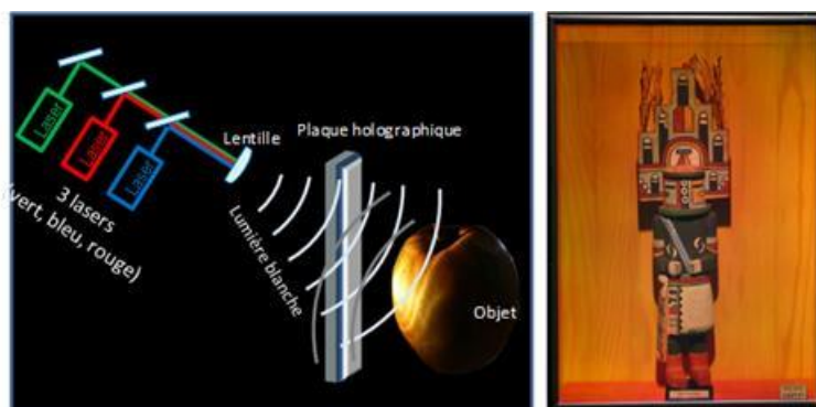
Figure 110. Expérience d'holographie en lumière blanche (gauche). Hologramme couleur restituable en lumière blanche (KACHINA HEMIS (statue indienne sud des états unis), Réalisation Y. Gentet)(droite).
