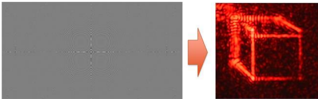
Figure 113. Exemple de l'hologramme d'un cube généré numériquement à Télécom ParisTech puis reconstitué par diffraction. On note un décalage de la face supérieure dû à une malencontreuse erreur de calcul !
