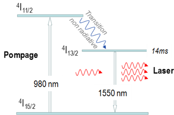
Figure 86. Système à 3 niveaux d'un amplificateur à fibre dopée erbium.
