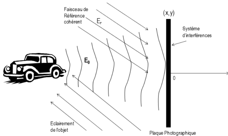
Figure 96. Schéma de principe de l'enregistrement d'un hologramme
