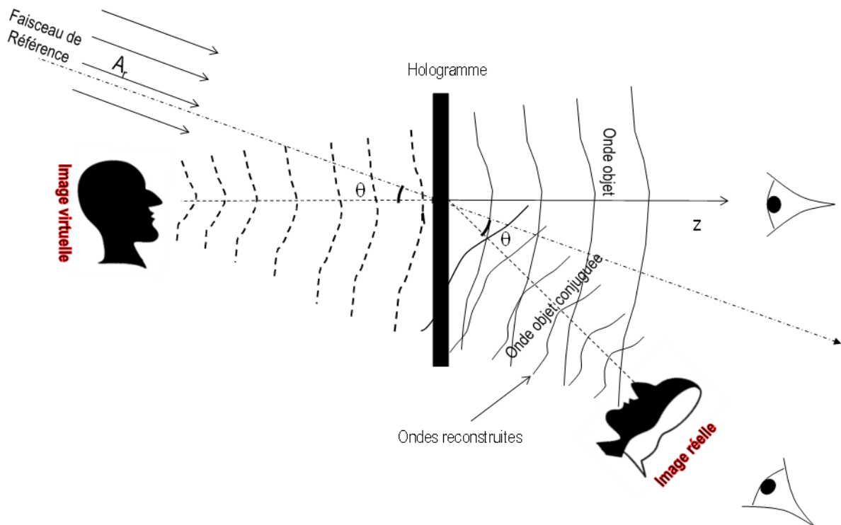
Figure 102. Relecture d'un hologramme hors-axe
