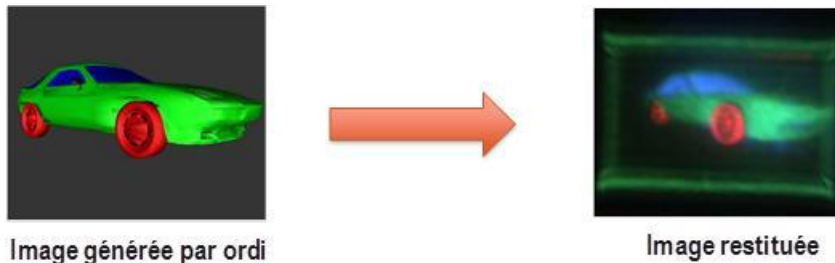
Figure 114. Exemple d'hologramme numérique généré par ordinateur et restituée par un modulateur spatial de lumière.
