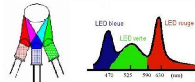
Figure 78. Diode blanche RVB : Génération de lumière blanche à l'aide de trois sources LED Rouge, Verte, Bleue
