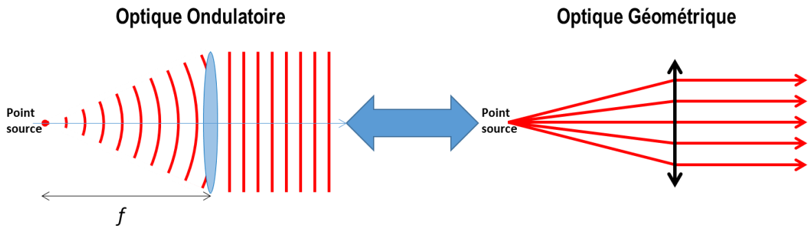
Figure 22. La lentille vue en optique géométrique (droite) ou en optique ondulatoire (gauche). Source ponctuelle dans le plan focal objet, sur l'axe optique.
