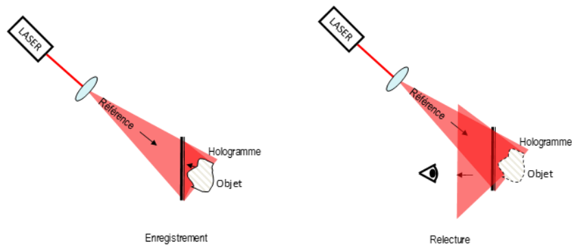
Figure 109. Enregistrement et relecture d'un hologramme en réflexion : l'hologramme de Denisyuk
