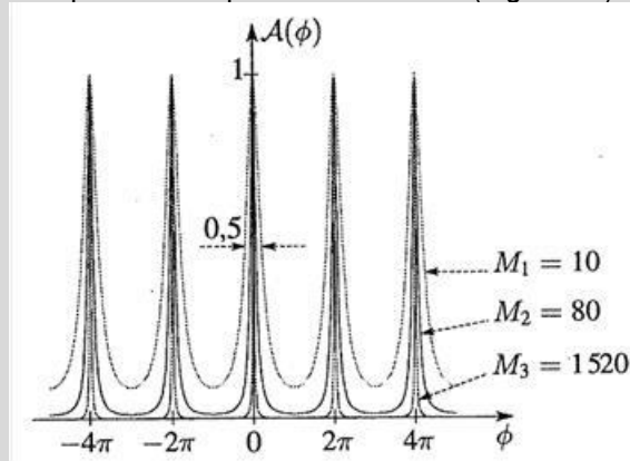
Figure 89. Fonction d'Airy pour différentes valeurs de M
