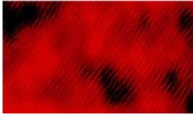
Figure 101. Photographie au microscope des franges d'interférences enregistrées sur un hologramme
