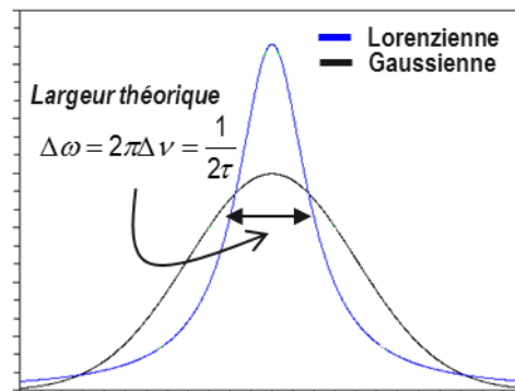
Figure 77. Spectre Lorentzien Théorique d'une émission lumineuse
