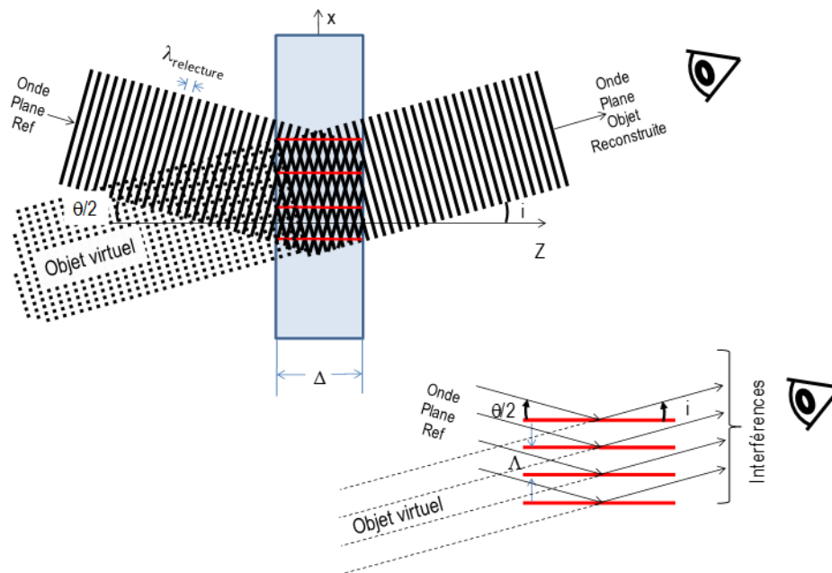
Figure 104. L'onde de référence est diffractée par le réseau de Bragg. Ceci permet de reconstruire l'objet. Si l'onde de référence est identique à l'onde de référence initiale (même longueur d'onde et même angle), alors i = \theta/2 .
