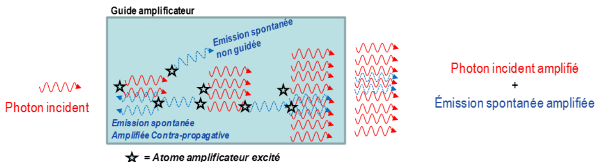
Figure 82. Principe détaillé de l'amplification dans un guide amplificateur
