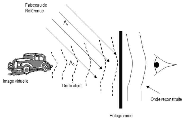
Figure 97. Reconstitution de l'onde objet par un hologramme
