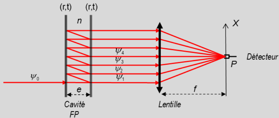
Figure 88. Interférences à ondes multiples dans une cavité Fabry-Perot. r_1 et r_2 sont les facteurs de réflexion en amplitude sur chaque miroir et t_1 et t_2 les facteurs de transmission correspondants. Remarque : toutes ces ondes sont en réalité superposées. Sur ce dessin, elle sont volontairement décalées pour faciliter la compréhension du phénomène.
