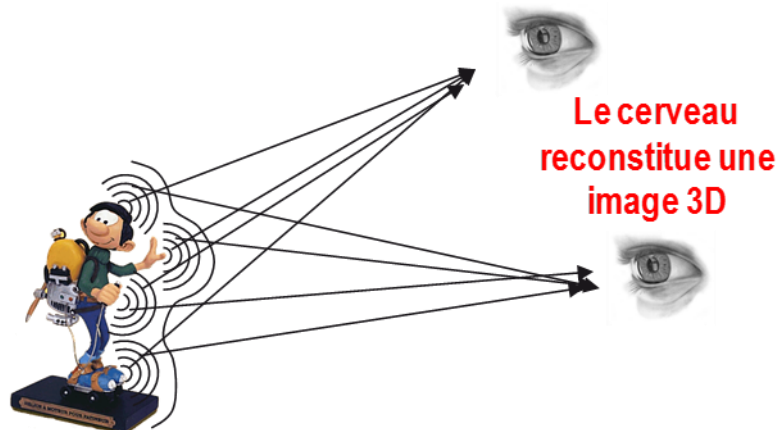
Figure 94. Principe de la vision volumique de l'être humain : la stéréoscopie
