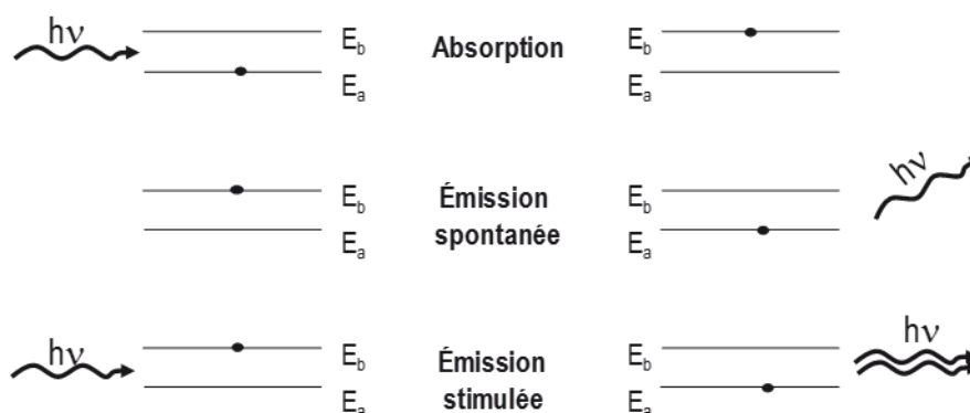
Figure 81. Schémas des transitions entre états
