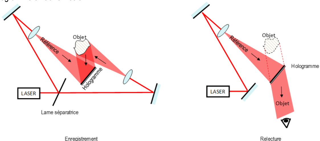
Figure 108. Enregistrement et relecture d'un hologramme en transmission.
