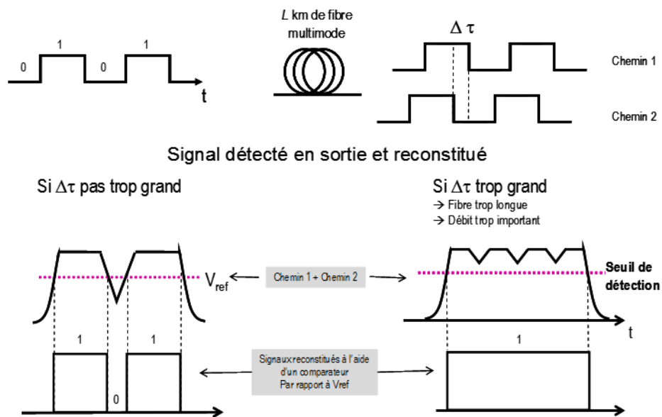
Figure 60. Reconstitution d'un signal dans une fibre multimodale
