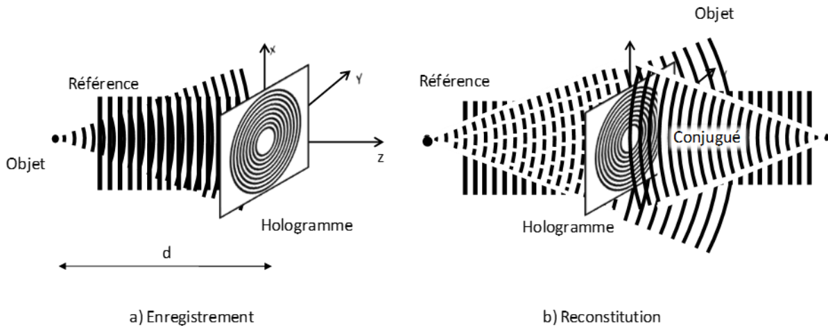
Figure 100. Hologramme d'une onde sphérique provenant d'un point source. L'onde conjuguée produit une image réelle du point source. L'onde objet produit elle une image virtuelle de ce point.
