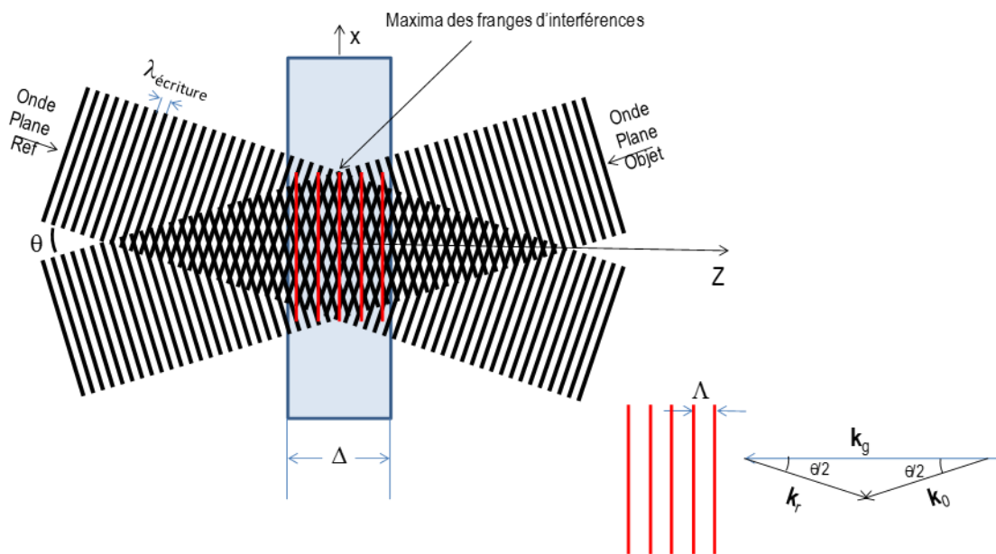
Figure 105. Un hologramme en réflexion est enregistré en plaçant le faisceau de référence et le faisceau objet de part et d'autre de la plaque holographique. Les franges d'interférences sont alors parallèles à la surface de la plaque holographique.
