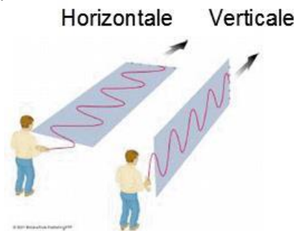
Figure 11. Illustration d'une polarisation rectiligne, verticale ou horizontale.
