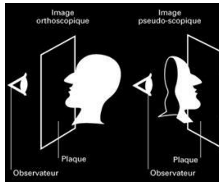
Figure 98. Différence entre une image orthoscopique et pseudoscopique
