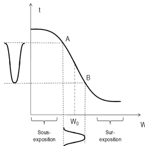
Figure 107. Facteur de transmission de la plaque en fonction de l'énergie reçue au moment de l'enregistrement.
