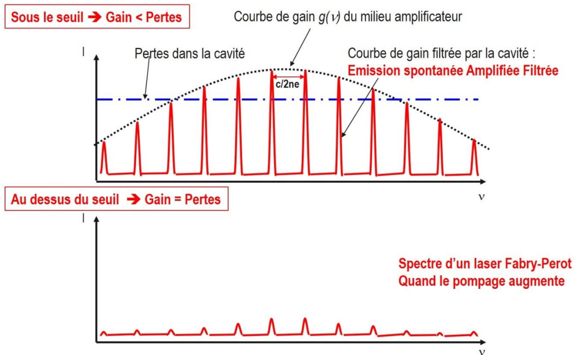
Figure 90. Résumé schématique du fonctionnement d'un laser
