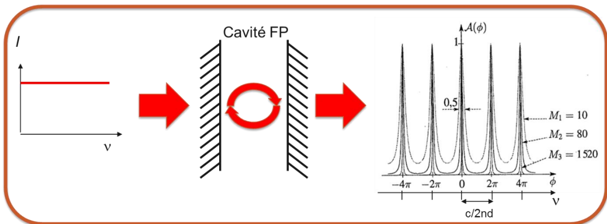
Figure 87. Transmission d'une cavité Fabry-Pérot en fonction de la fréquence.
