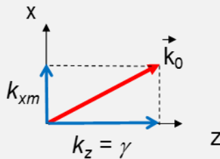
Figure 67. Constantes de propagation des ondes guidées. \|\vec{k}_0\| = 2\pi/\lambda
