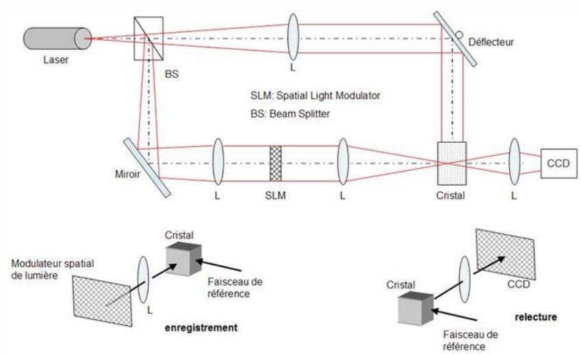
Figure 112. Principe de base de la mémoire holographique
