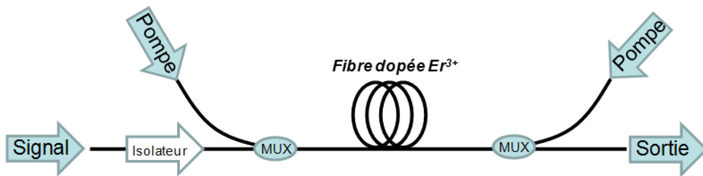
Figure 84. Représentation schématique d'un EDFA
