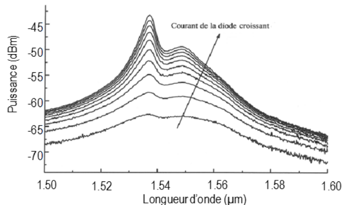
Figure 80. Spectre d'émission d'une source à fibre dopée à l'Erbium.
