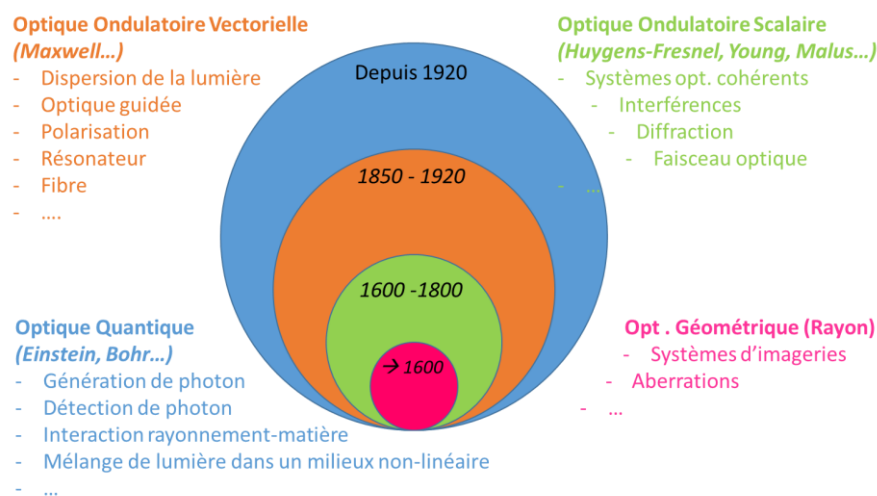
Figure 1. Historique des différentes théories optiques. Le cadre de ce cours se situe en optique ondulatoire scalaire .
