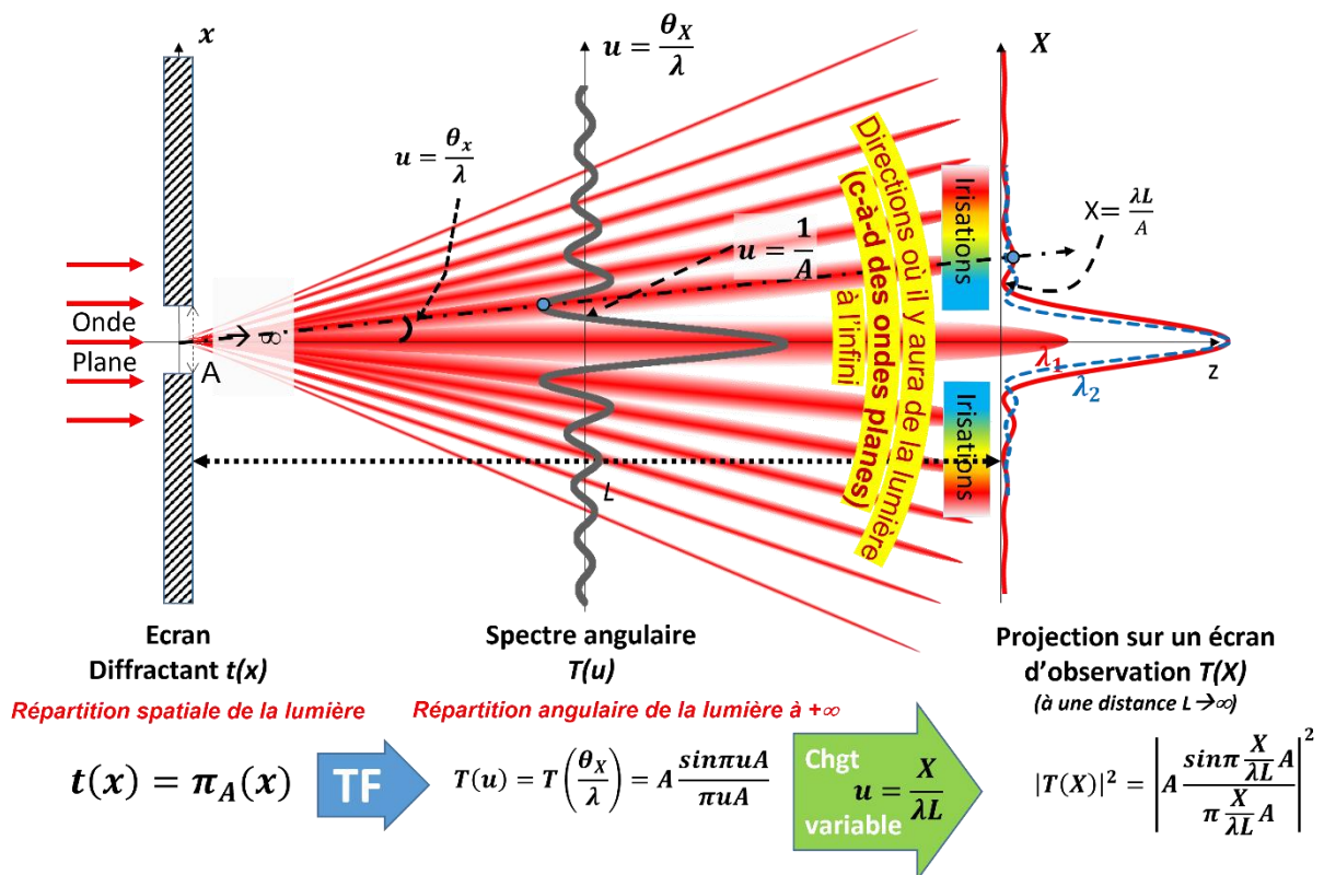
Figure 38. Illustration de la diffraction de Fraunhofer d'une ouverture carrée éclairée par une onde plane
