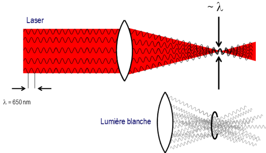
Figure 91. Propriété de cohérence spatiale d'un faisceau laser.
