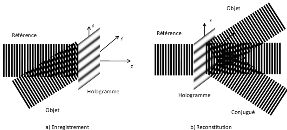
Figure 99. L'hologramme d'une onde plane oblique est un réseau de diffraction sinusoidal.
