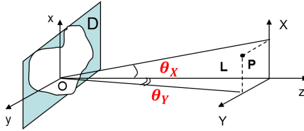
Figure 37. Lien entre angles et fréquence angulaires
