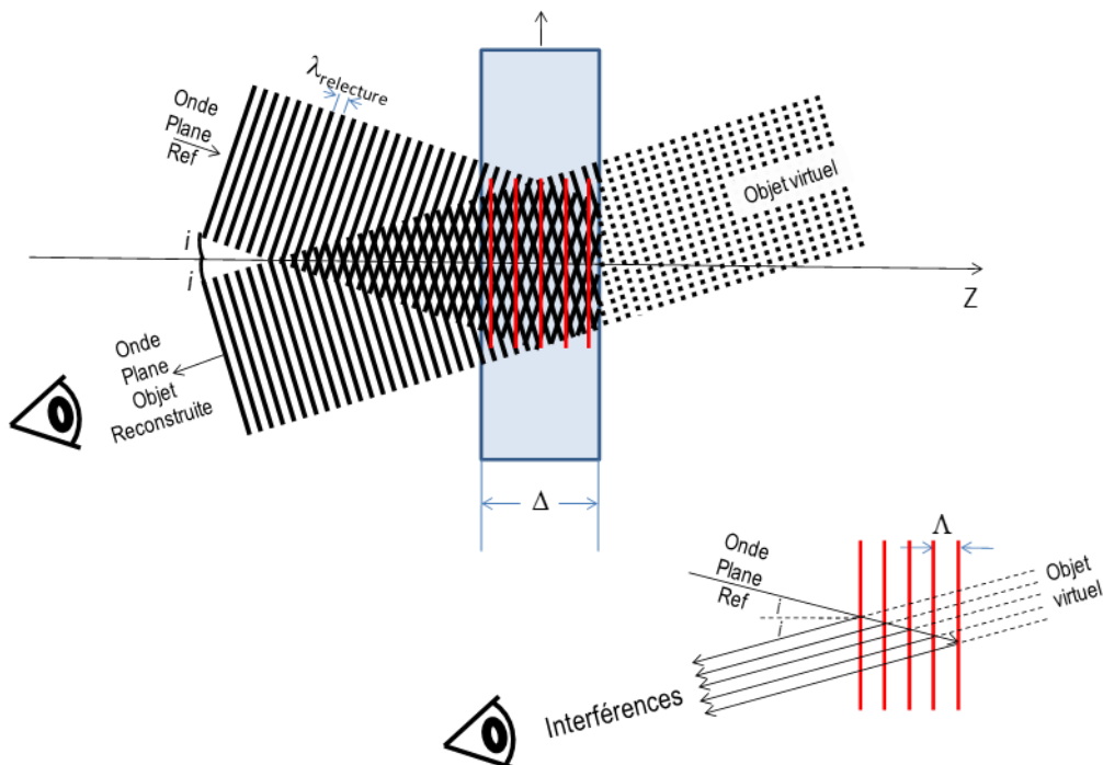
Figure 106. Reconstruction d'un hologramme en réflexion. La méthode d'enregistrement permet d'inscrire simultanément l'hologramme ainsi qu'un filtre de Bragg permettant de relire l'hologramme en lumière blanche.
