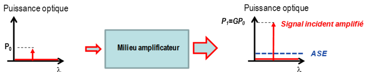
Figure 83. Principe macroscopique de l'amplification dans un guide amplificateur de gain G
