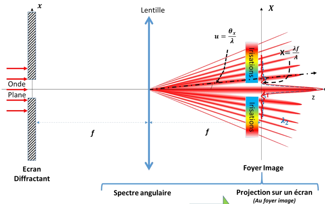
Figure 40. Diffraction par une lentille convergente : Spectre angulaire
