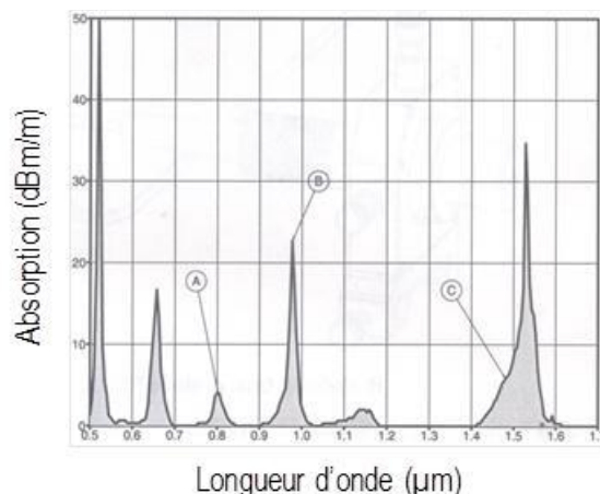
Figure 85. Spectre d'absorption d'une fibre dopée à l'Erbium. A : Bande autour de 800nm. B : Bande autour de 980. C : Bande autour de 1480nm
