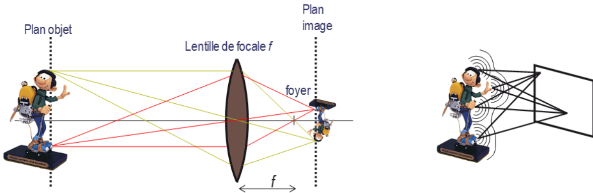
Figure 95. Principe de la formation d'une image (gauche). Enregistrement d'une image sans lentille (droite): chaque point de l'objet éclaire l'intégralité du plan image, la plaque est éclairée de manière (quasi) uniforme, il n'y a pas d'image.
