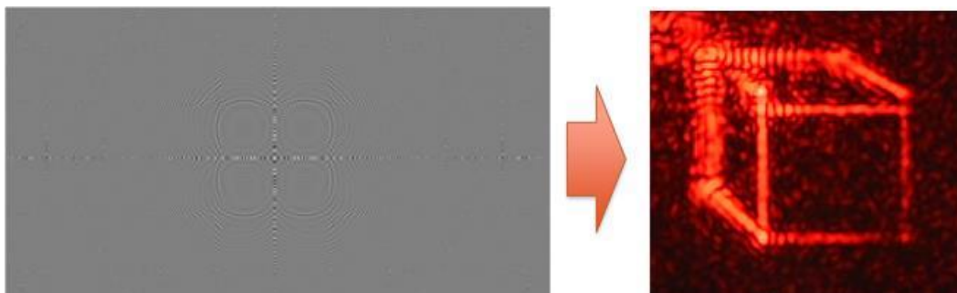
Figure 113. Exemple de l'hologramme d'un cube généré numériquement à Télécom ParisTech puis reconstitué par diffraction. On note un décalage de la face supérieure dû à une malencontreuse erreur de calcul !
