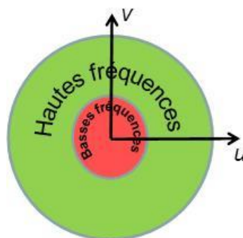
Figure 49. Notion de hautes et basses fréquences spatiales dans le plan de diffraction
