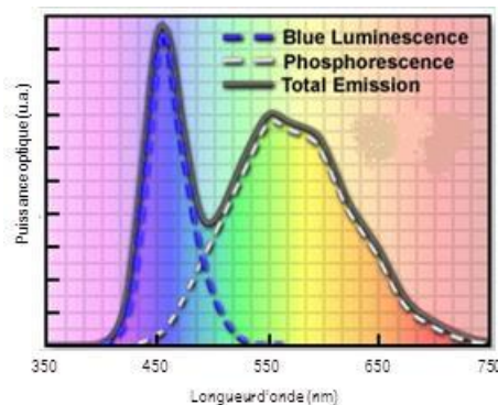
Figure 79. Spectre d'émission d'une LED blanche émise par une diode bleue couplée à du phosphore ré-émettant dans le jaune.
