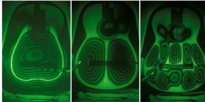
Figure 111. Image holographique des vibrations d'une guitare. Les lignes les plus claires sont les lignes nodales i.e. les endroits où il n'y a pas de vibration.
