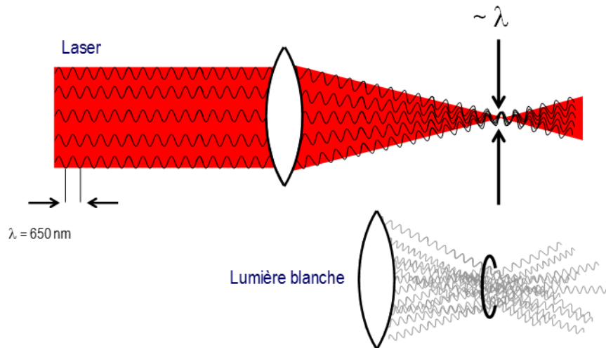
Figure 91. Propriété de cohérence spatiale d'un faisceau laser.
