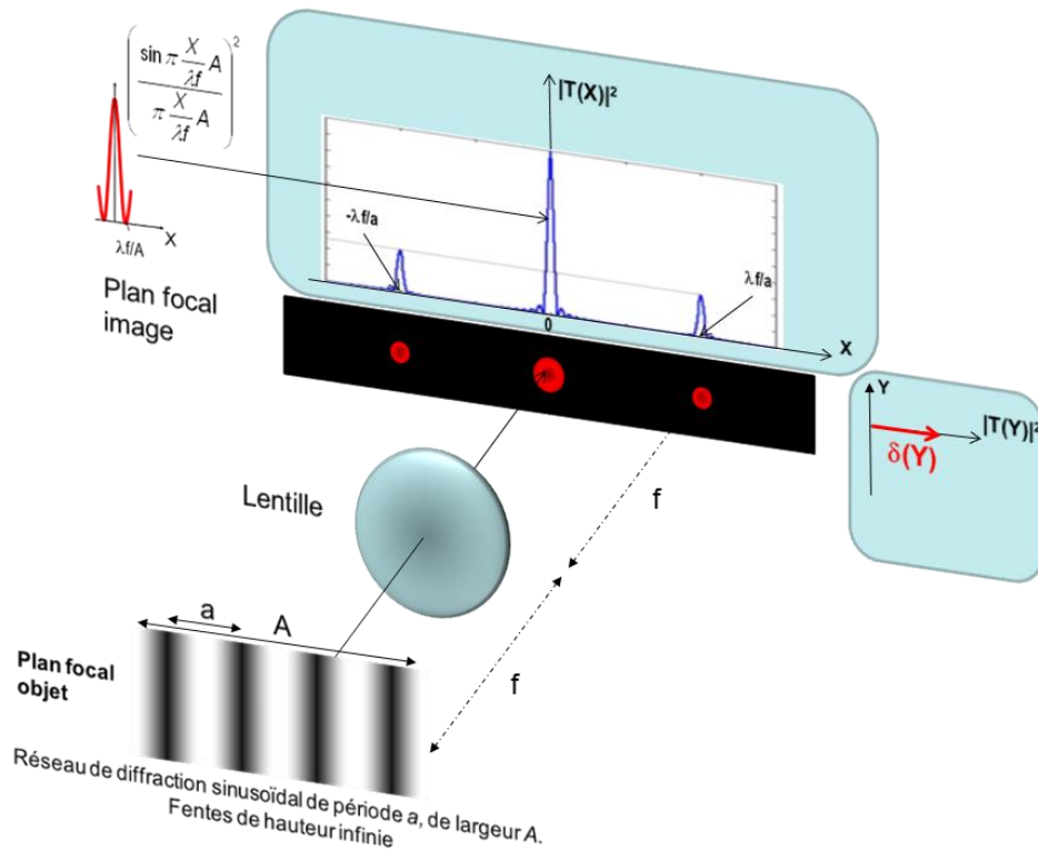
Figure 47. Diffraction par une lentille convergente d'un réseau sinusoidal tronqué spatialement.
