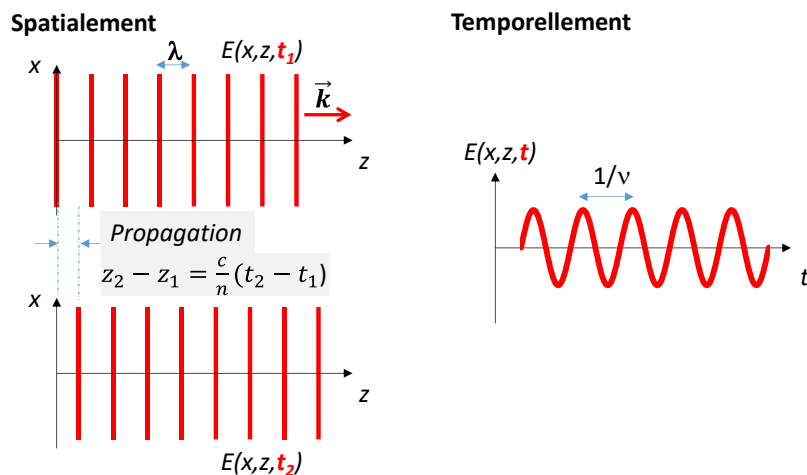
Figure 14. Une onde plane se propageant dans la direction z est une fonction périodique de z avec une période spatiale \lambda et une fonction périodique de t avec une période temporelle 1/v .
