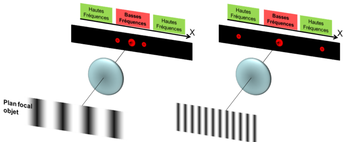
Figure 48. Influence du pas du réseau sur la figure de diffraction. Lien entre les variations d'amplitude de l'image et les fréquences spatiales
