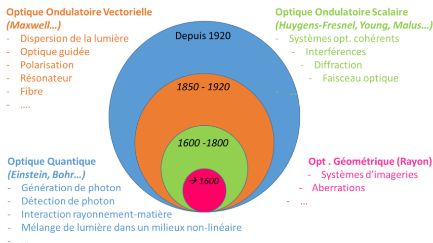
Figure 1. Historique des différentes théories optiques. La cadre de ce cours se situe en optique ondulatoire scalaire .
