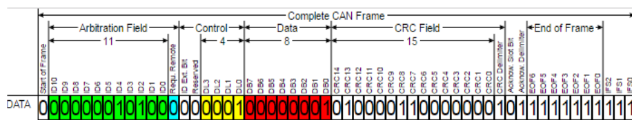
Un paquet CAN Data (1 octet de donnée)
