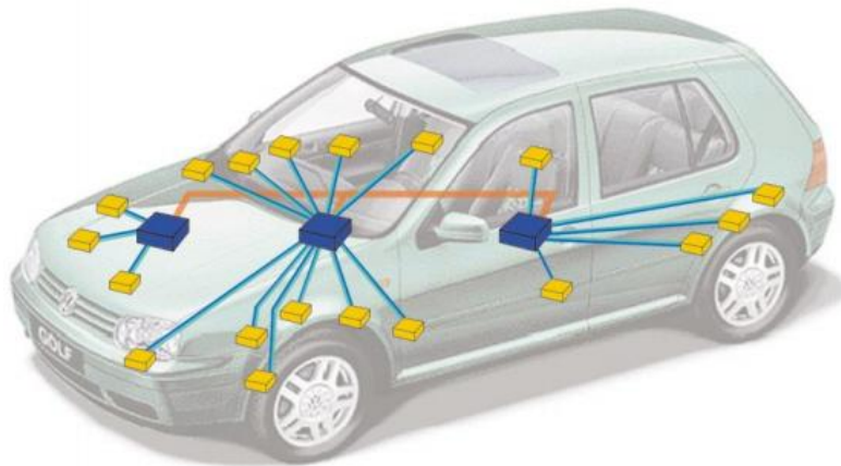
Exemple d'un véhicule comportant trois ECUs et un BUS CAN
