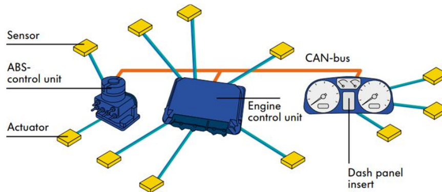
Exemple de CAN-bus reliant trois ECUs
