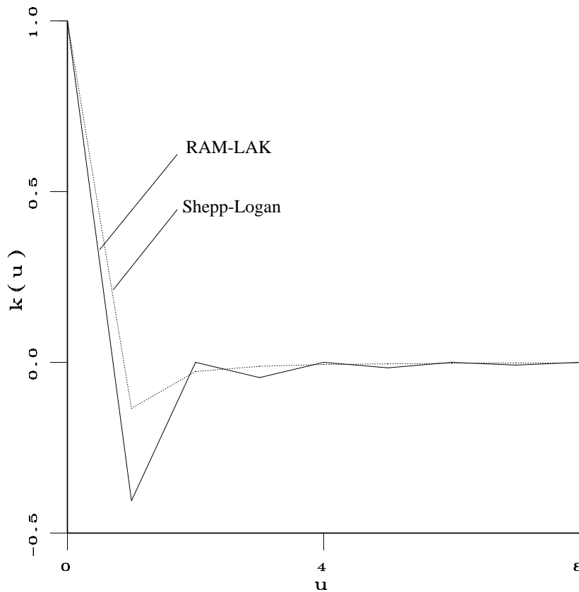
FIG. 8 – Filtres numériques (RAM-LAK et Shepp-Logan).
